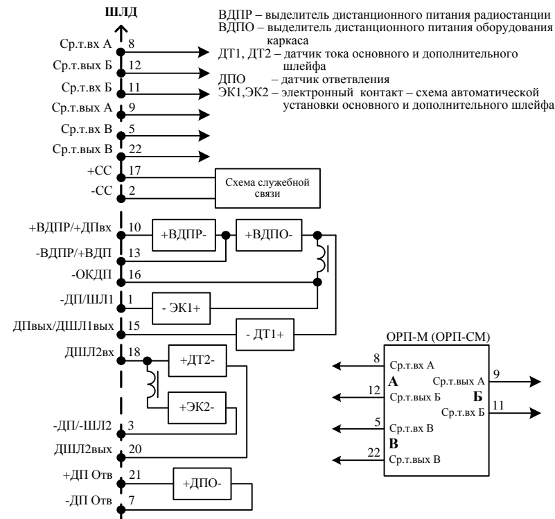
Рисунок а) – Организация цепей дистанционного питания в каркасах ОРП-М, ОРП-СМ
