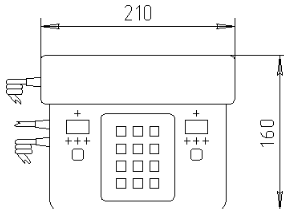
Рисунок А.4 - Пульт ПДС-М
