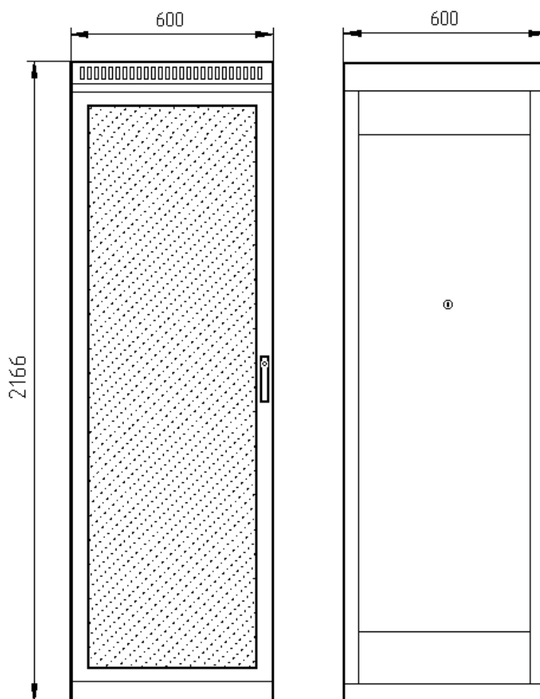
Рисунок А.1 - Каркас СЛЮД-М
