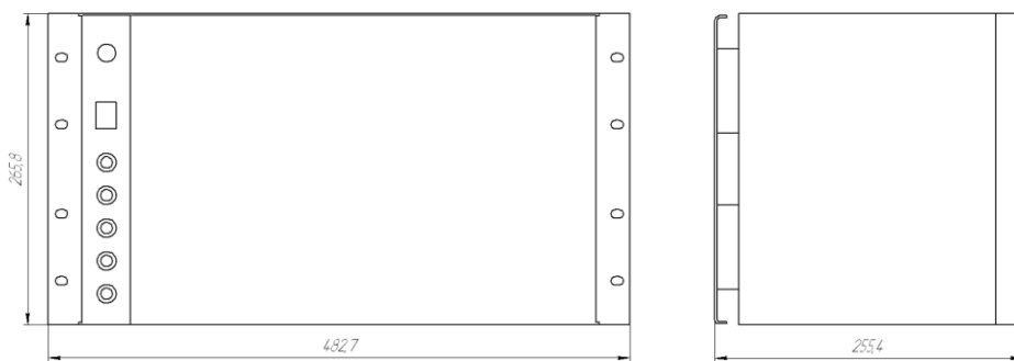
Рисунок А.14 - Каркас ОРП-СМ
